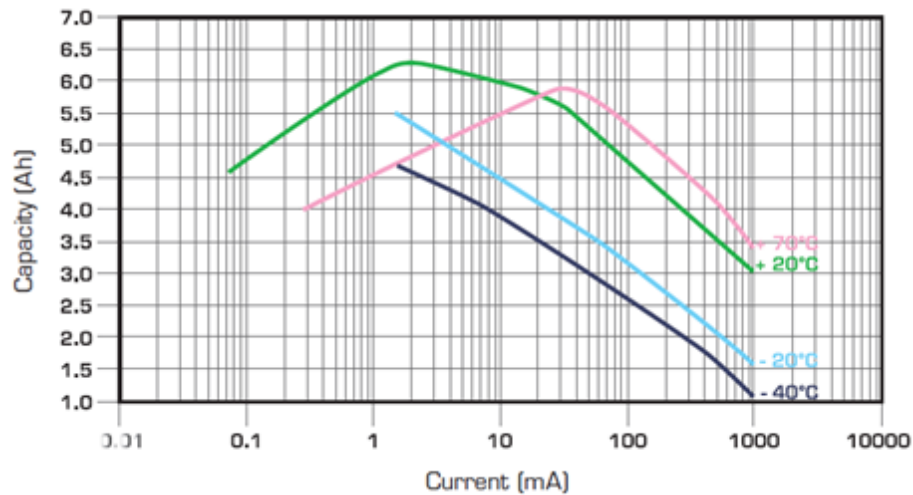
Зависимость ёмкости от рабочего тока и температуры
